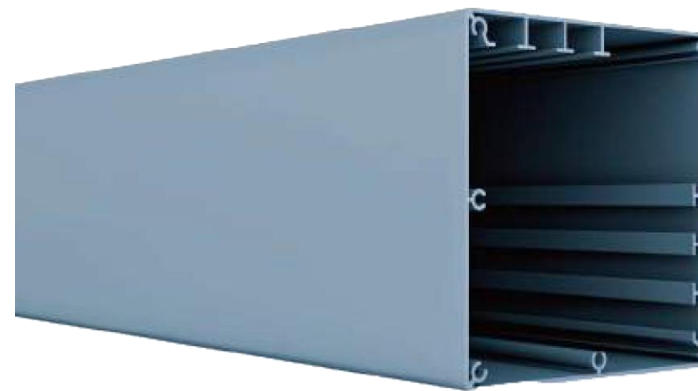
Column size: 150*150mm; Optional size: 180*180mm; Profile thickness: 2.0mm
